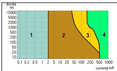
Zone di pericolosità della corrente elettrica continua
