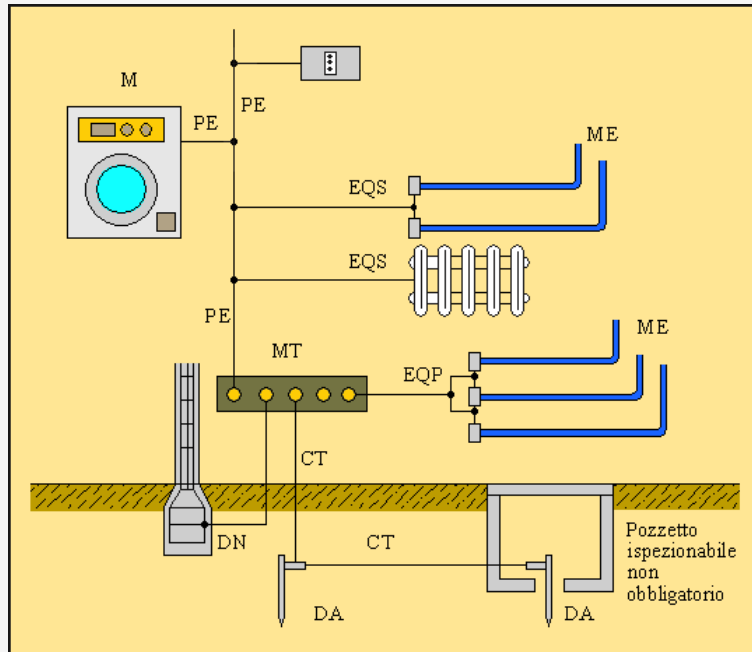
Elementi fondamentali di un impianto di terra
