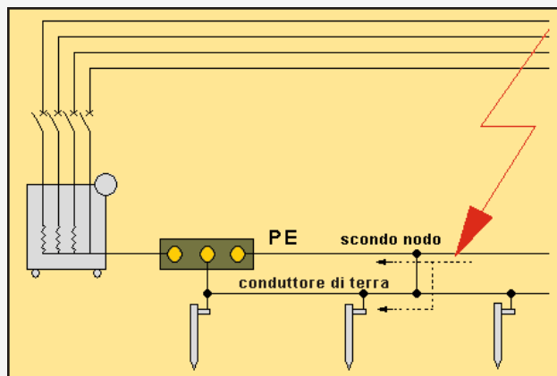
Il conduttore di terra può essere interessato da una frazione della corrente di guasto solo se esistono più nodi equipotenziali
